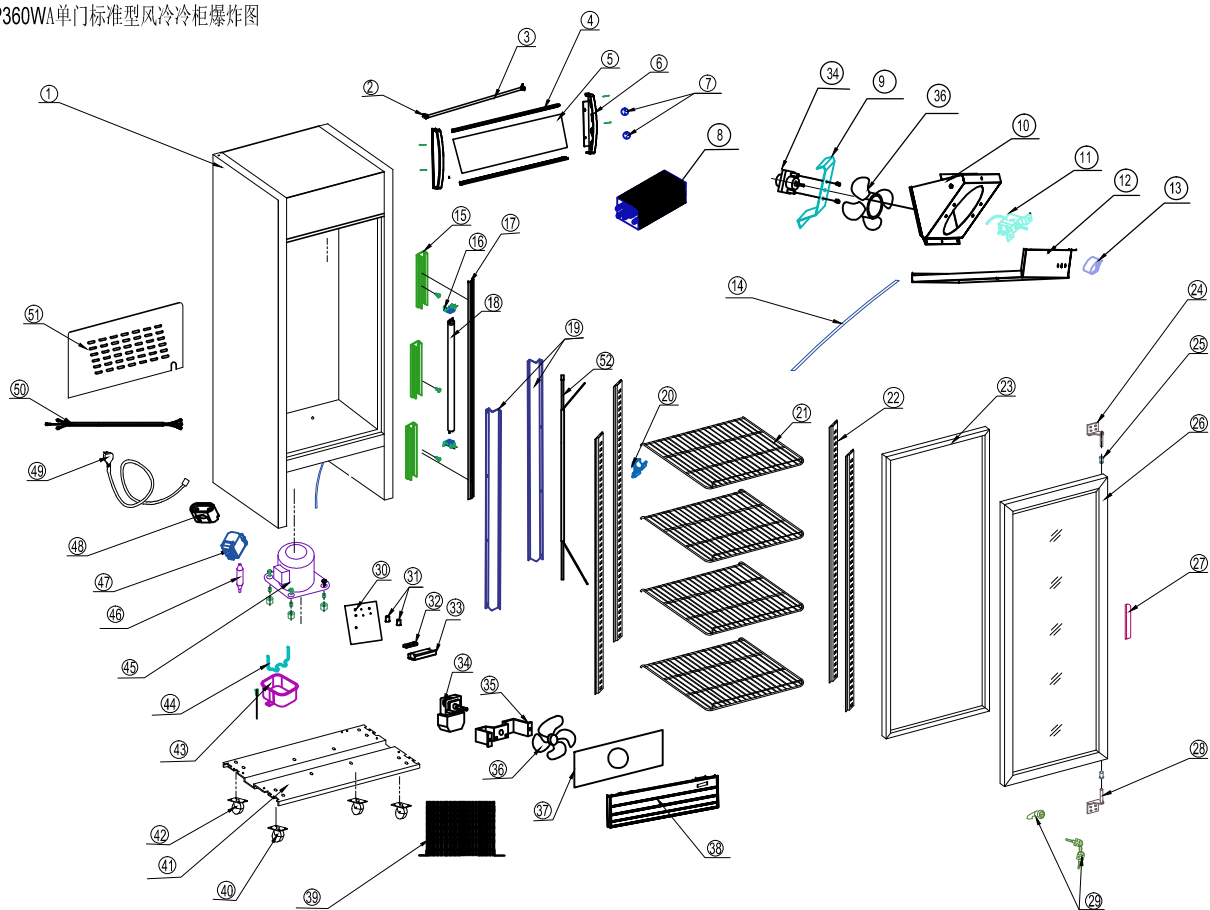
SS-P360WA单门标准型风冷冷柜爆炸图
