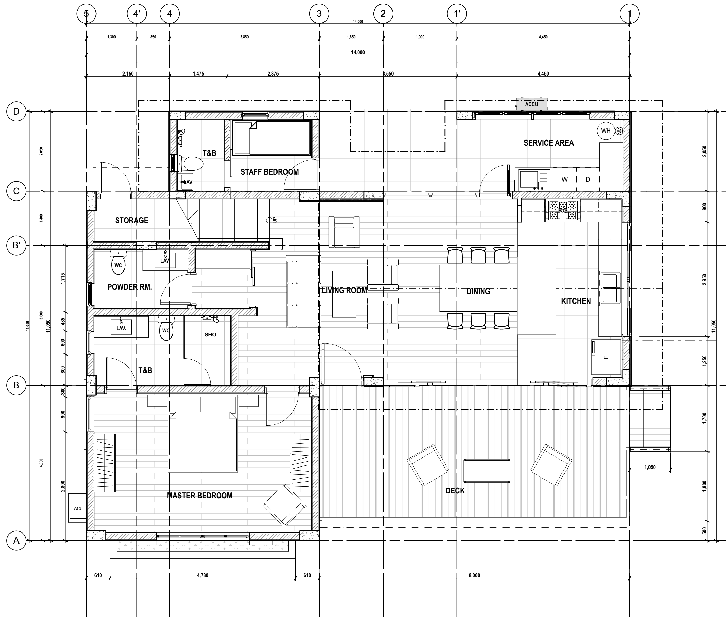
1 A-102 1/F FURNITURE LAYOUT SCALE: 1:50
