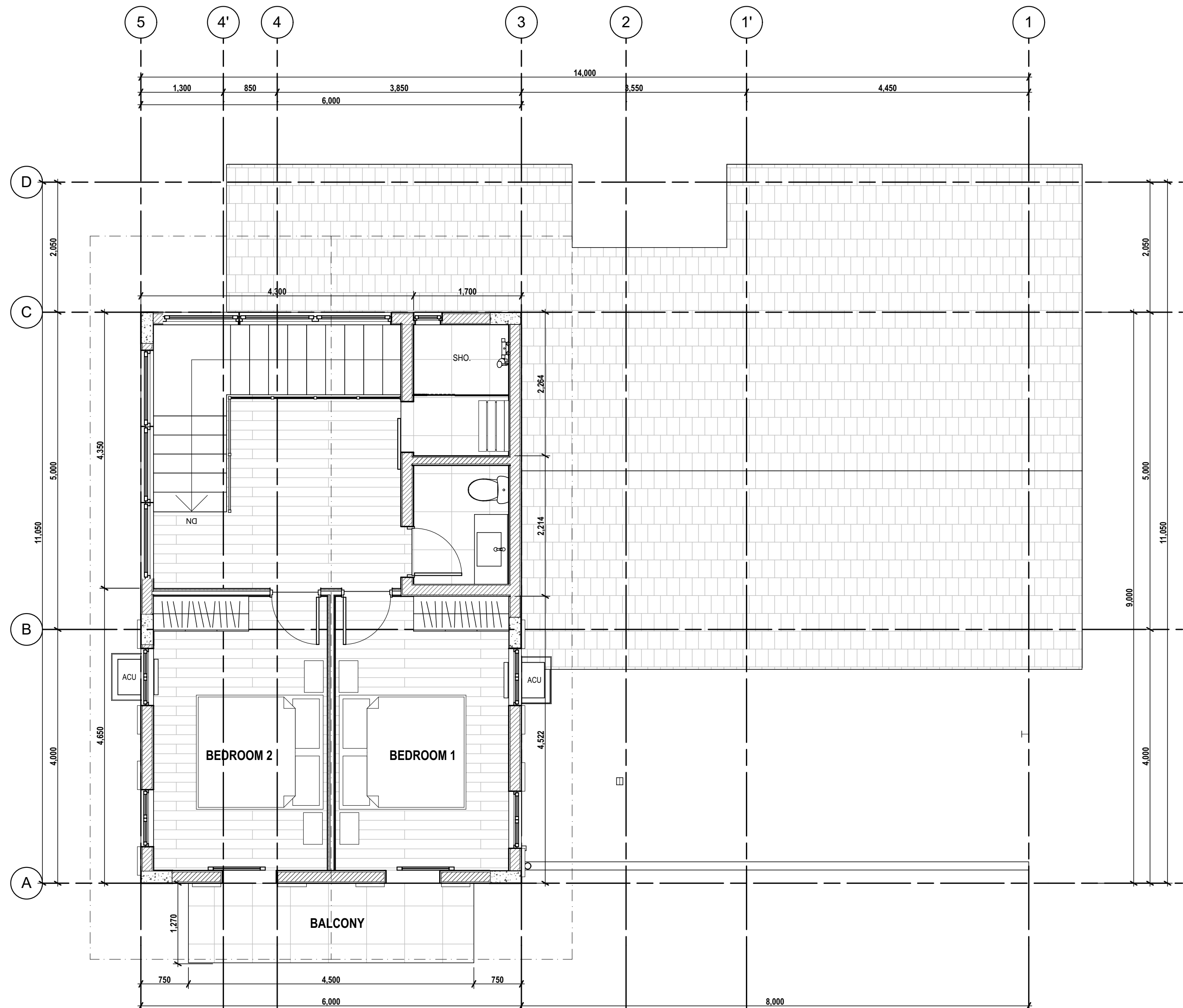
2 A-102 2/F FURNITURE LAYOUT SCALE: 1:50
